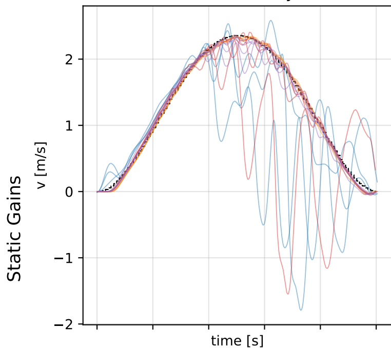
linear velocity
